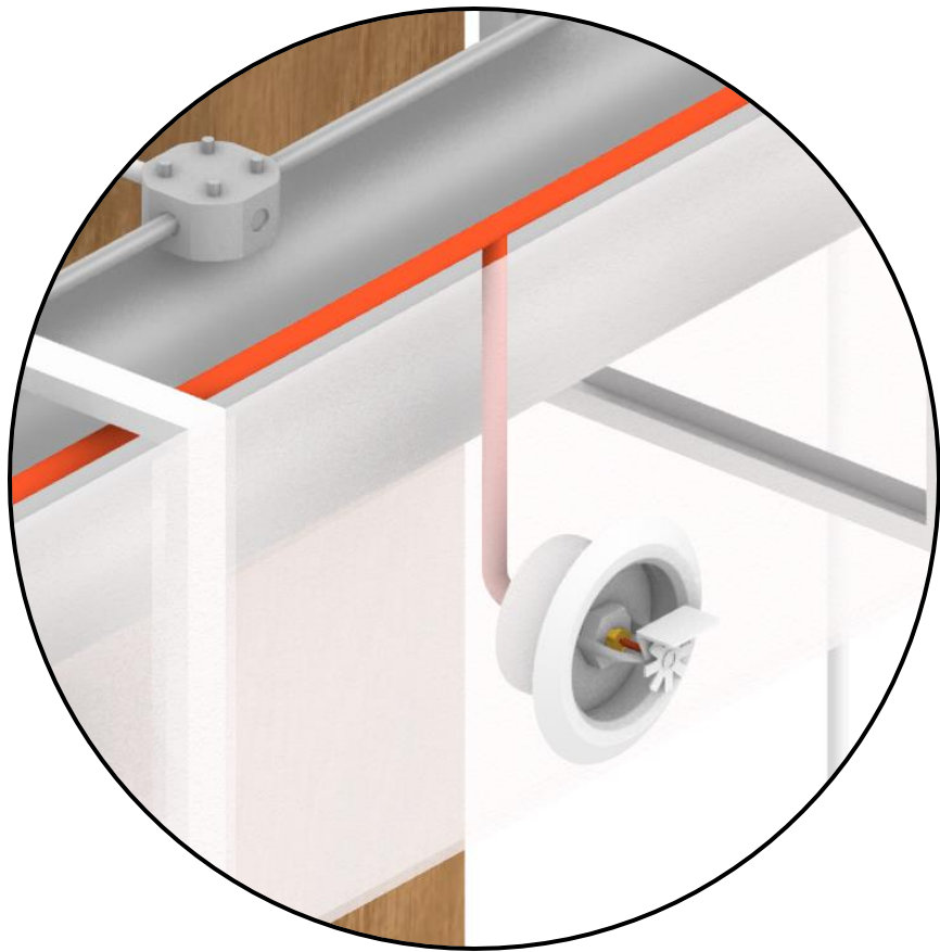
Sprinkler
